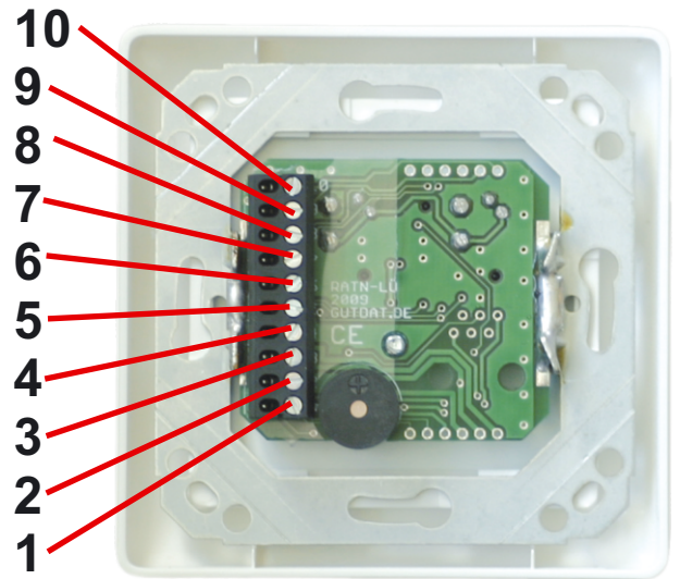
Abbildung: ZSL ohne Elektronikmodul
